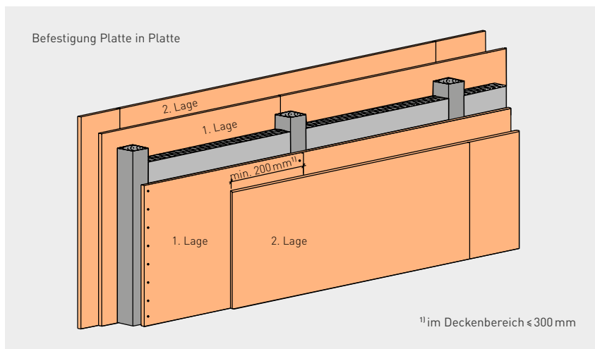
Abstand und Verbrauch von Befestigungsmitteln bei Wänden und Decken mit fermacell® Gipsfaser-Platten bei der Befestigung Platte in Platte – Befestigung der 1. Plattenlage wie bei Wand/Dach oder Decke (vgl. S. 101/103) Holz 1-lagig
