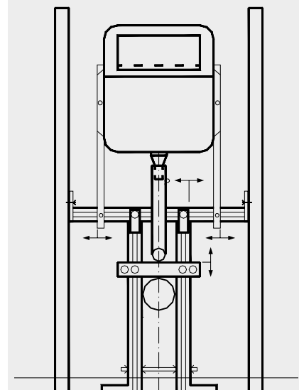
Tragständer für wandhängende WCs mit Einbauspülkästen
