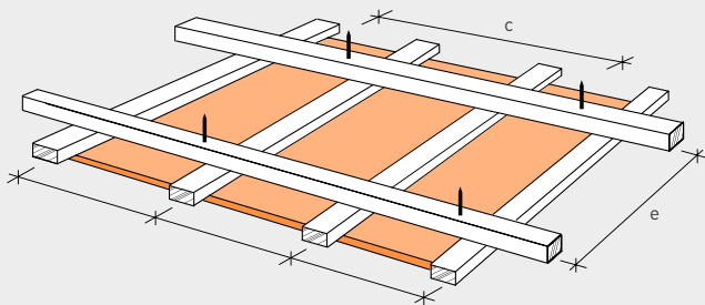
Grundlatte, direkt befestigt
