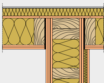
Beispiel Gebäudeklasse 4: Objektbezogene Detaillösung zum Anschluss fermacell Außenwand (F 90-B/K 2 30 innen -K 2 60 außen ) fermacell Brandwand (F 90-B/K 2 60)
