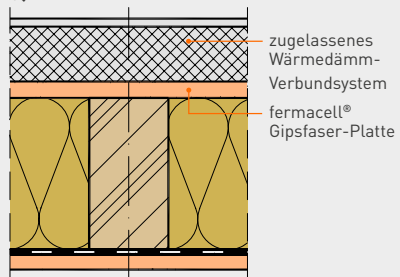
Wirksamer Wetterschutz WDVS
