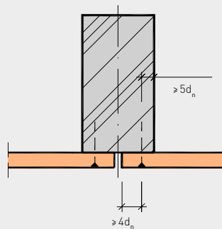
Bild 6: Abstände bei einer Mittelrippe/Nägeln
