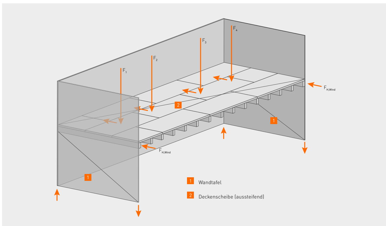
Lasteintrag (Wind) aus Deckenscheibe in seitliche Wandtafeln
