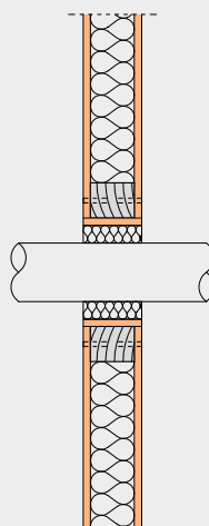
Rauchrohrdurchführung
