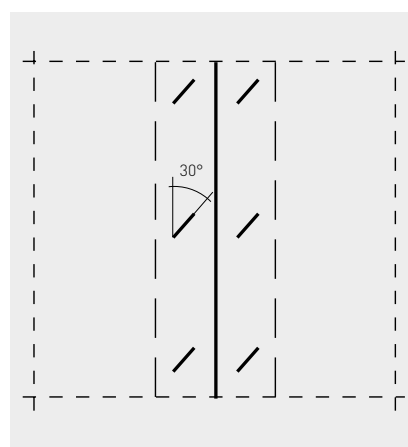
Einschlagwinkel der Klammern
