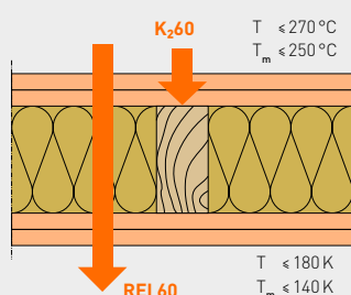
Beispiel Gebäudeklasse 4: Ausführung einer Holzständerwand (REI 60/K 2 60) gemäß den Anforderungen der Muster-Richtlinie (M-HFH HolzR)/hochfeuerhemmendes Bauteil
