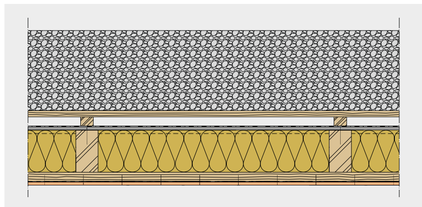
Aufbau 22 HD 12 Sonderlösung F 30-B – fermacell® Powerpanel HD Reetdach
