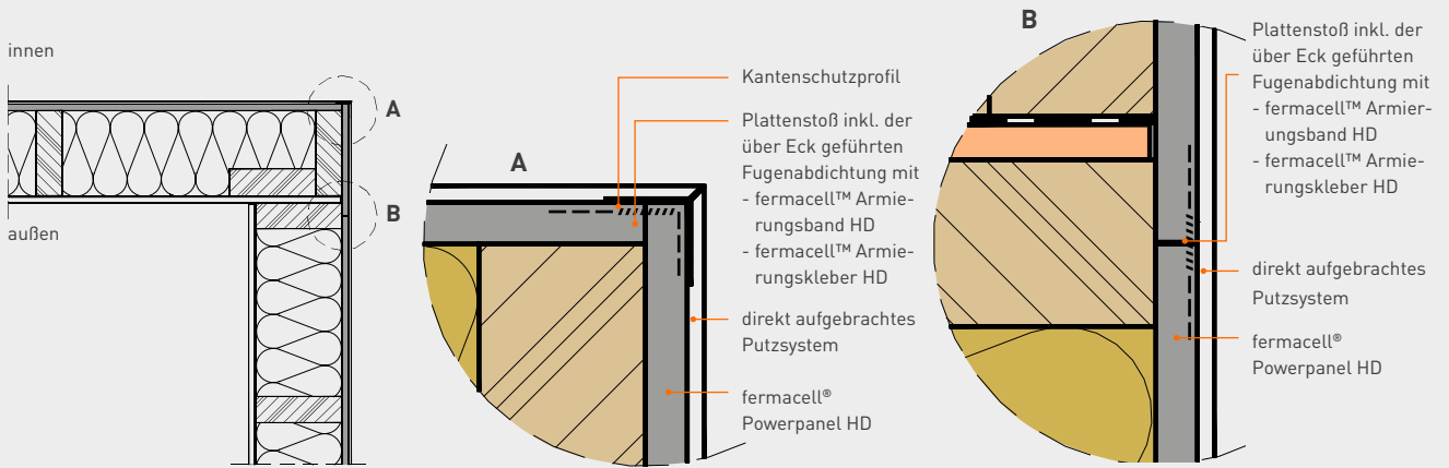
Ausbildung einer Außenecke mit der fermacell® Powerpanel HD Platte
