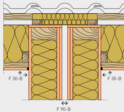
Beispiel Gebäudeklasse 1-3: Ausführung von Übergängen zwischen trauf- und giebelständigen fermacell Gebäudeabschlusswänden
