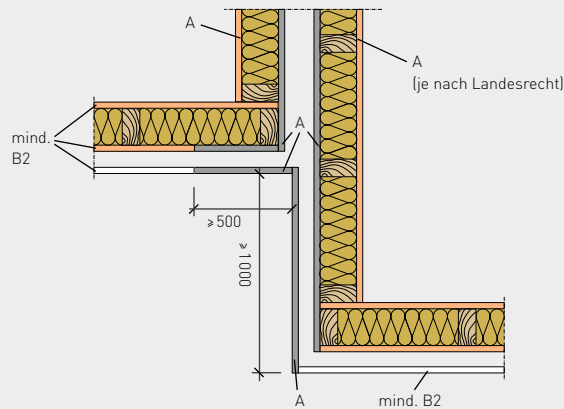
Beispiel Gebäudeklasse 1-3: Ausführung von nichtbrennbaren Bekleidungen - versetzte Bauweise
