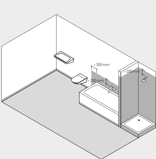
Häusliches Bad mit Wanne und Dusche
