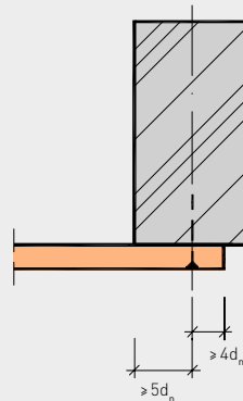
Bild 8: Abstände bei einer Randrippe/Nägeln
