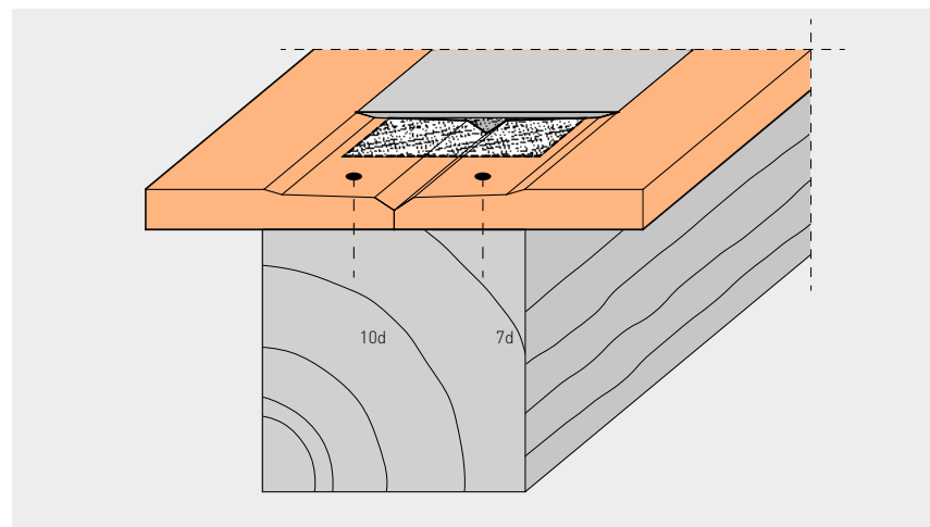
Randabstände TB-Kante für Nägel
