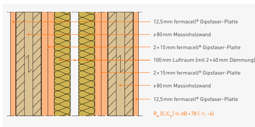
Gebäudeabschlusswand – tieffrequenter Einsatz (Beispiel)
