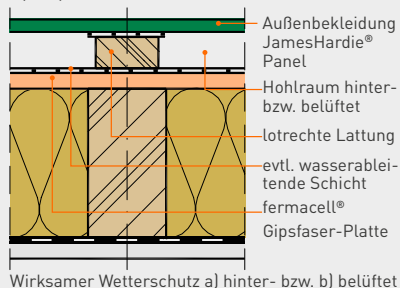
Wirksamer Wetterschutz a) hinter- bzw. b) belüftet
