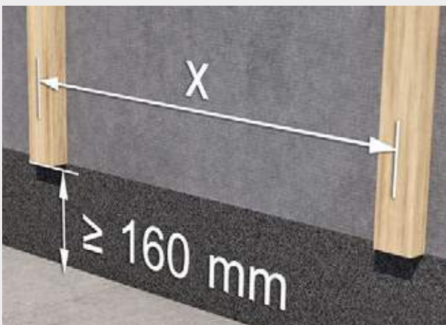
Abstand zur Unterkante der Traglattung entsprechend Bauvorschriften, jedoch mindestens 160 mm.
