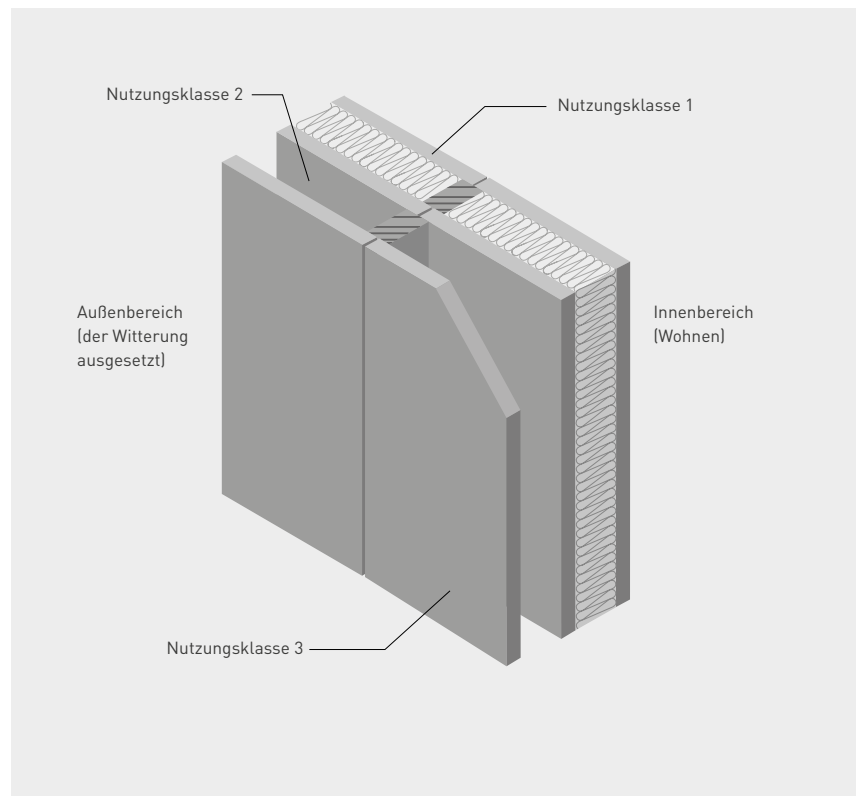
Definition der Nutzungsklassen gemäß DIN EN 1995-1-1
