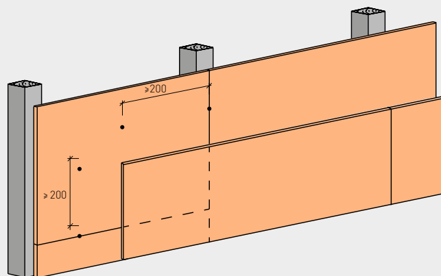
Versetzen der zweiten Lage bei mehrlagiger Beplankung
