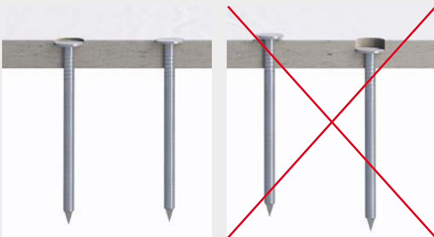
Befestigungsmittel bündig mit Oberfläche oder max. 1 mm versenkt eintreiben.
