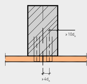
Bild 7: Abstände bei einer Mittelrippe/Klammern
