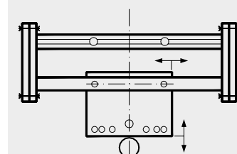
Traverse für leichte Handwaschbecken
