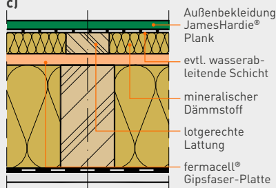
Wirksamer Wetterschutz nicht belüftet
