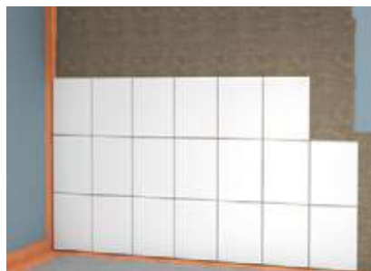
Abb. 5: Sicherstellung der Abdichtung für die Wasser- einwirkungsklasse W0-I. Verfliesung mit fermacell™ Flexkleber im Dünnbettverfahren
