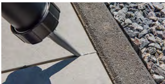
Schritt 1: Sopro Solitär® TF mit Silikonspritze im Überschuss in die Fuge einbringen
