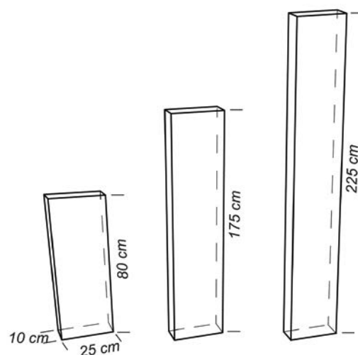
Technische Zeichnung der Palisaden
